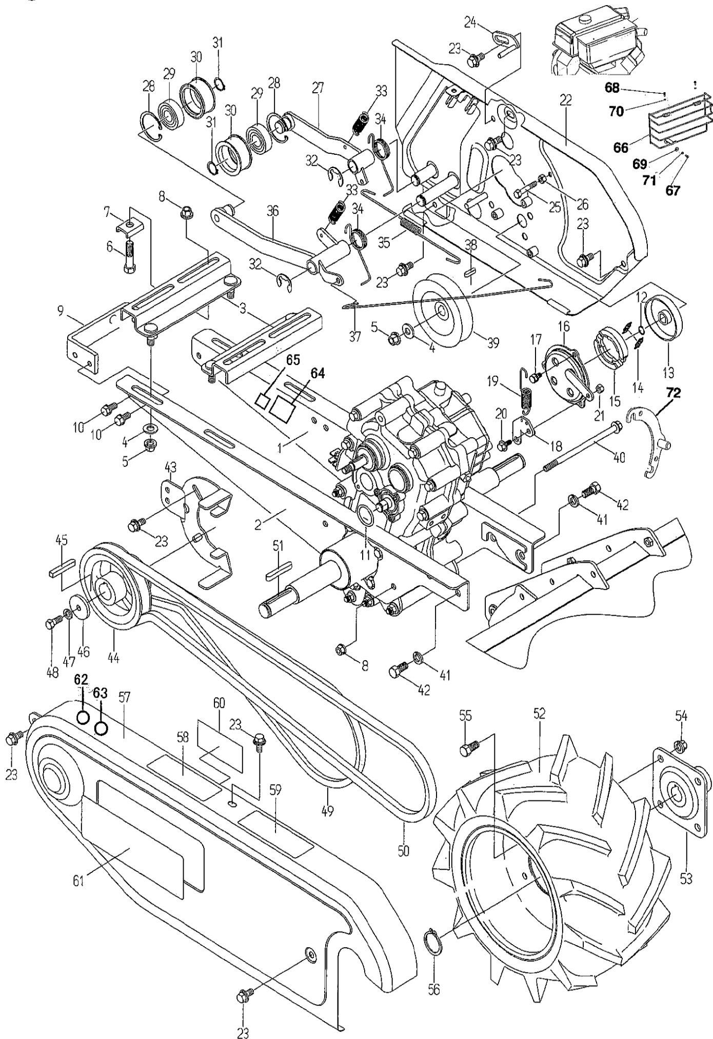
Fig. 3 FRAME
