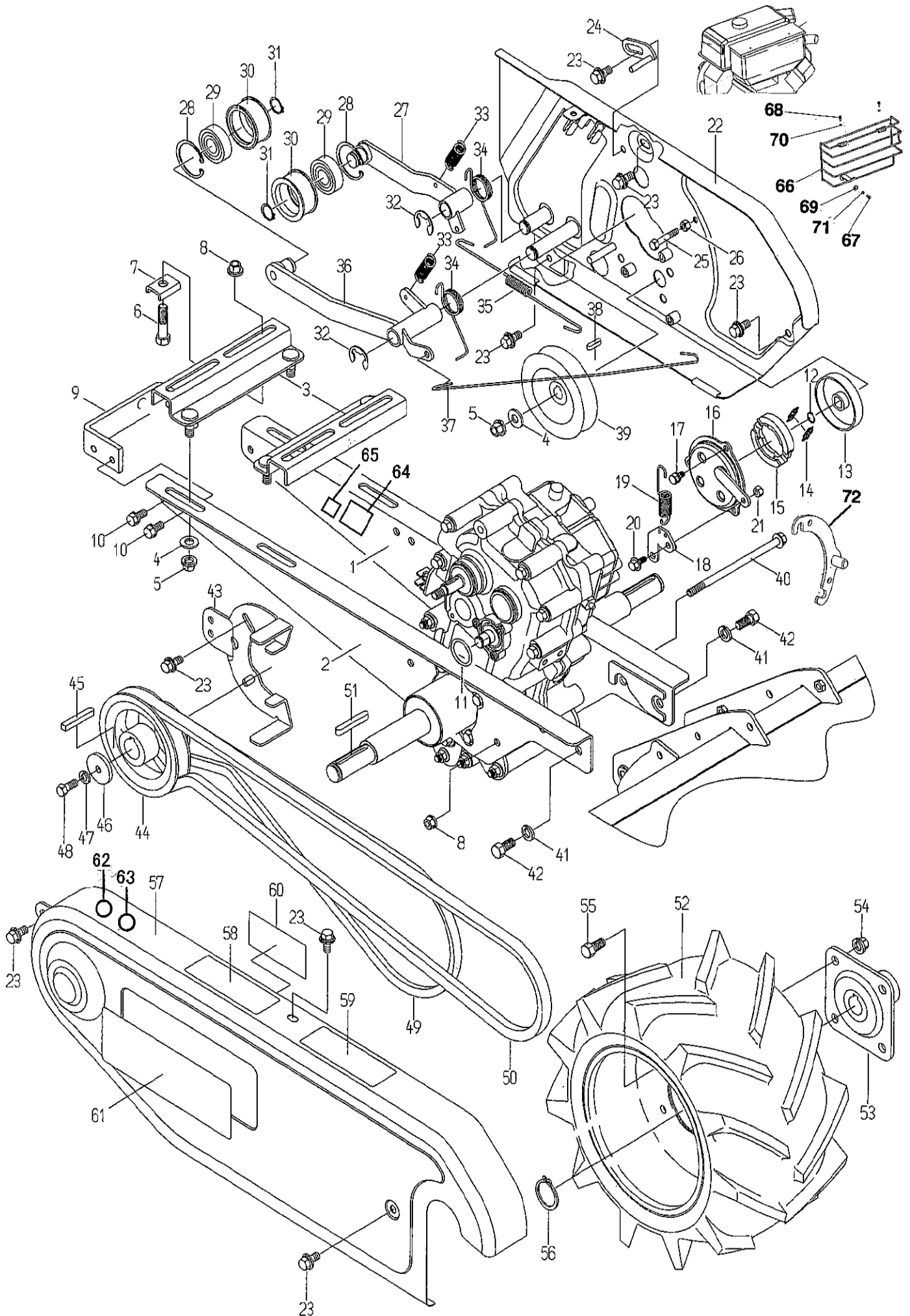
Fig. 3 FRAME
